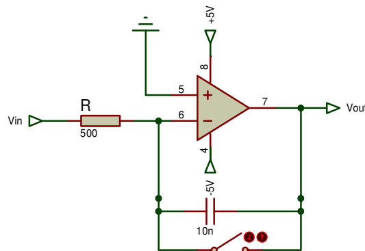
Fig. 6. Integrator
